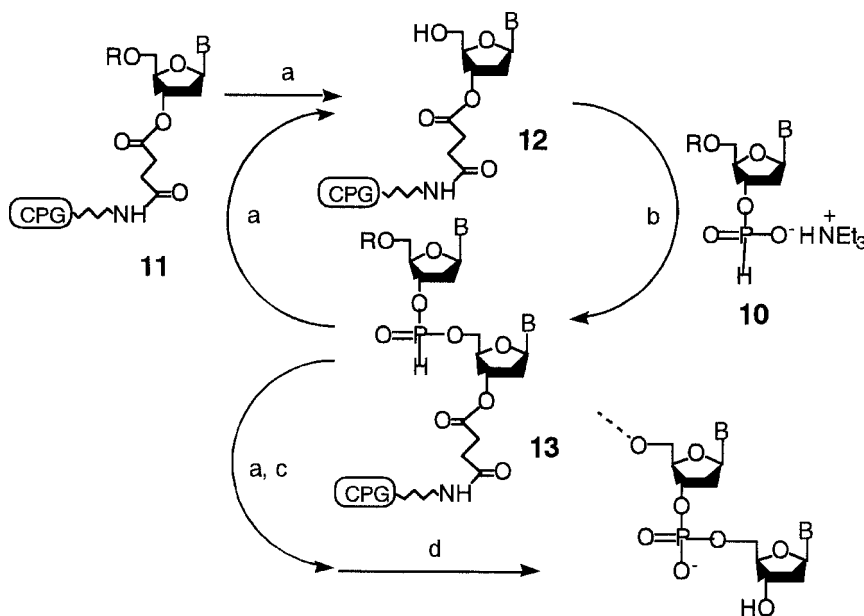
Scheme 5. Conditions (a) 1) 0.5 M \text{NH}_2\text{NH}_2\cdot\text{H}_2\text{O} , 2:3:5 \text{CH}_3\text{CO}_2\text{H} -pyridine- \text{CH}_3\text{CN} , 15 min, 2) 0.5 M imidazole, \text{CH}_3\text{CN} , 5 min, (b) 0.05 M 10 , 0.25 M pivaloyl chloride, 1:1 pyridine- \text{CH}_3\text{CN} , r.t., 10 min, (c) 3% \text{I}_2 , \text{H}_2\text{O} -19% pyridine-76% THF, r.t., 10 min, (d) conc. \text{NH}_4\text{OH} , r.t., 3 h and 55^\circ\text{C} , 6 h.
